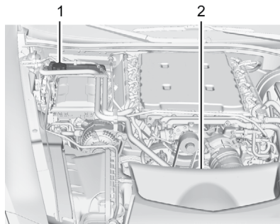
Двигатель LT4 с масляным резервуаром двигателя с сухим картером
